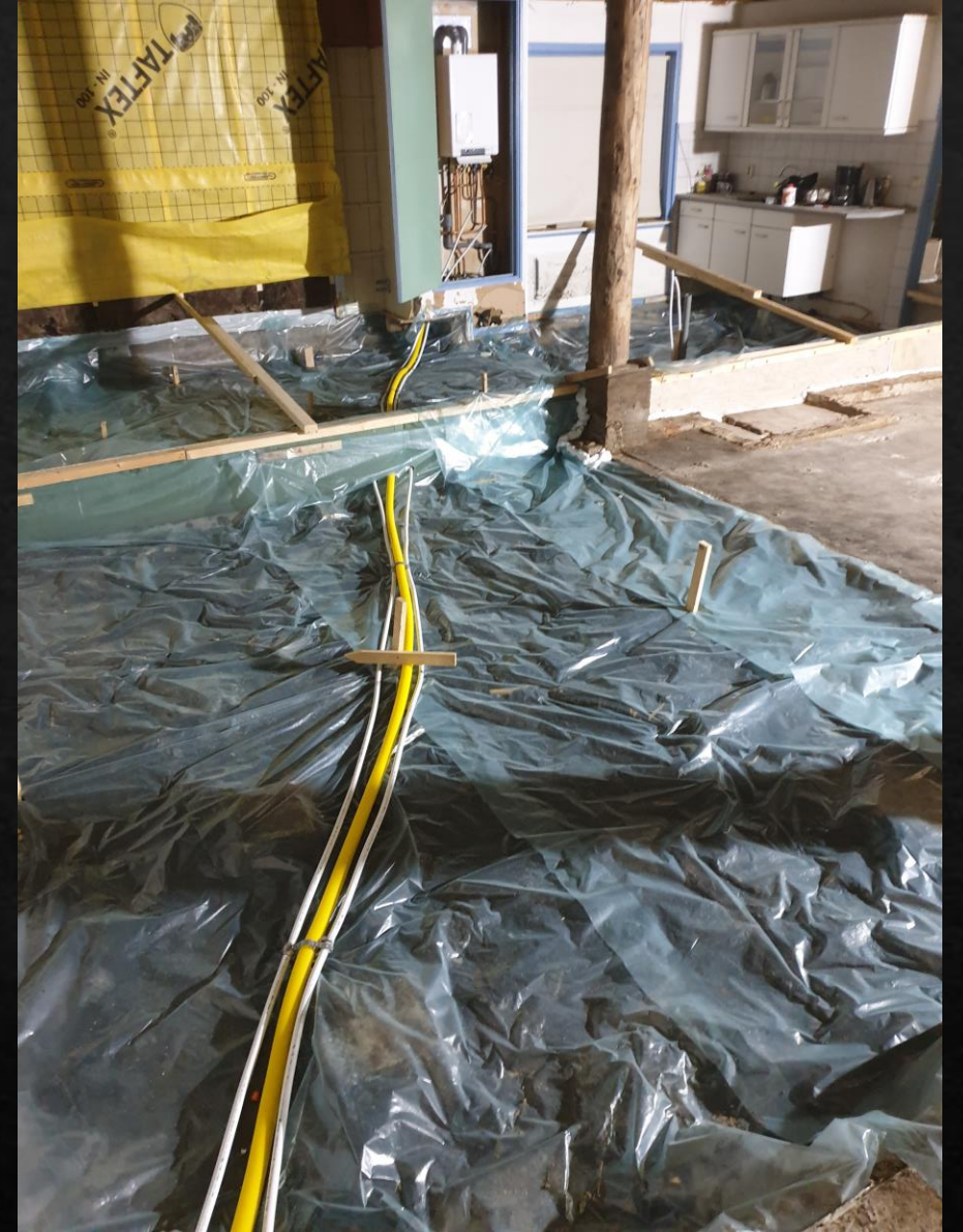
De vloer klaarmaken voor het schuimbeton
